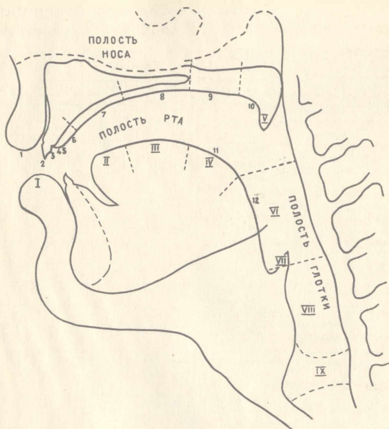
Рис. СХЕМАТИЧЕСКИЙ САГГИТАЛЬНЫЙ РАЗРЕЗ РЕЧЕВОГО АППАРАТА
