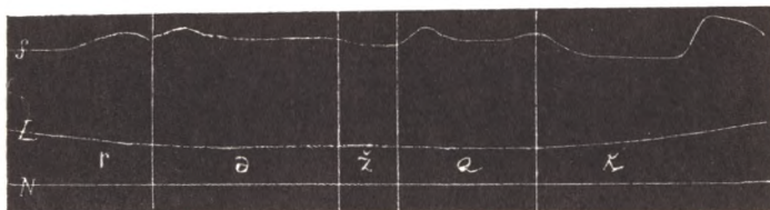
Фиг. 65. рыжакъ [rəʒak].
