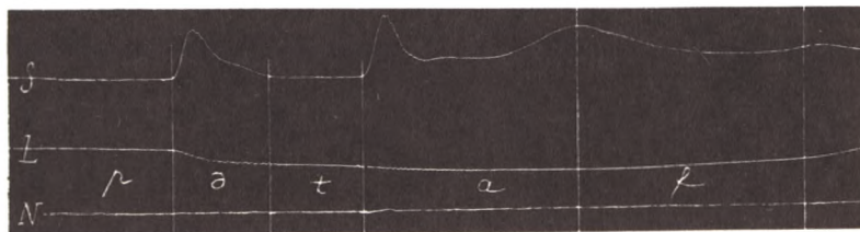
Фиг. 67. пытавъ [pətaf].
