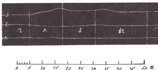
Фиг. 31. Носы [пласы]. Внизу масштабъ, который приблизительно годится для всѣхъ аналогичныхъ кривыхъ *), кромѣ фиг. 69.
