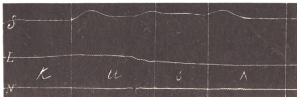
Фиг. 52. куса [kusa].
