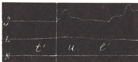
Фиг. 66. тюль [t'ul'].
