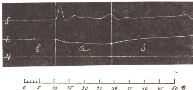
Фиг. 49. bas [bas]. Маштаб годится болѣе или менѣе для всѣхъ кривыхъ этого рода (кромѣ фиг. 69).
