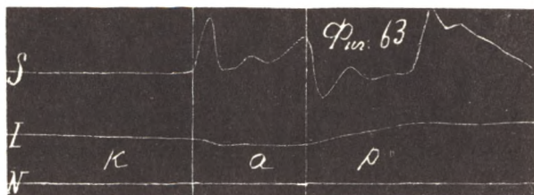
Фиг. 63. kap [kap], см. таблицу IV.
