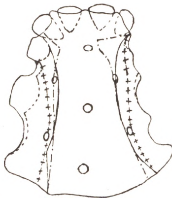
Фиг. 26. Сплошная линия—[i]; прерывистая—[i]; крестиками—[i].
