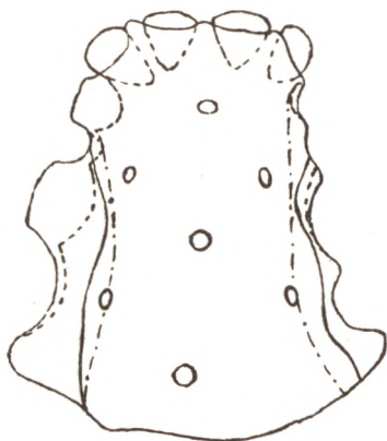
Фиг. 42. Сплошная линия— [ь]; прерывистая— [i-].
