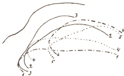
Фиг. 19. 1—[a]; 2—[e]; 3—[i]; 4—[ɔ]; 5—[u]; 6—[ы].
