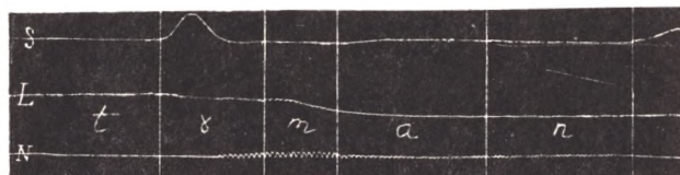
Фиг. 34. Туманъ [tsman].
