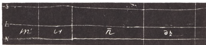
Фиг. 33. Минный [m' i - n: əb].
