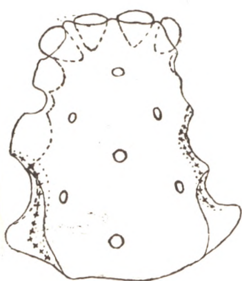
Фиг. 21. Сплошная линия — мы ; пунктирь — пыфз ; крестиками — пыпф .
