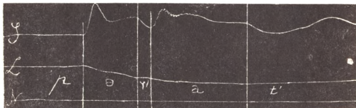
Фиг. 62. пырять [pə'at'].
