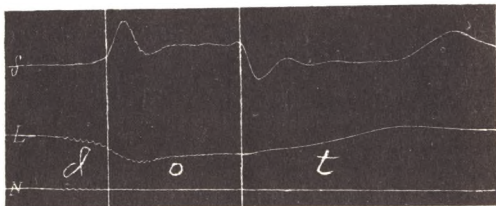
Фиг. 55. ётѡ (iotѡ) [jot].
