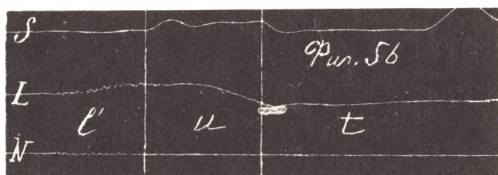
Фиг. 56. лютѡ [l'ut].
