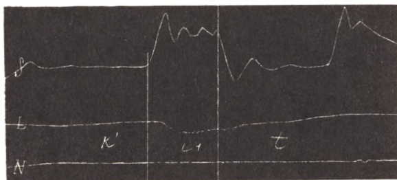
Фиг. 64. kita [ki-ti].
