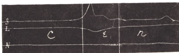
Фиг. 32. Цѣнѣ [сѣн].
