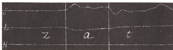
Фиг. 54. задъ [zat].
