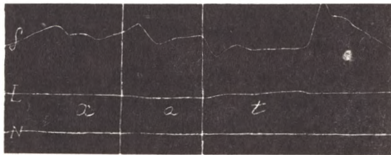
Фиг. 60. хатъ [xat], см. таблицу IV.
