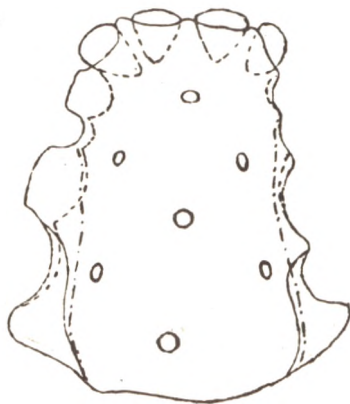
Фиг. 22. Сплошная линия — [ы]; прерывистая — [е-і-і]
