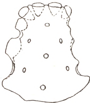
Фиг. 41. По бобу.
