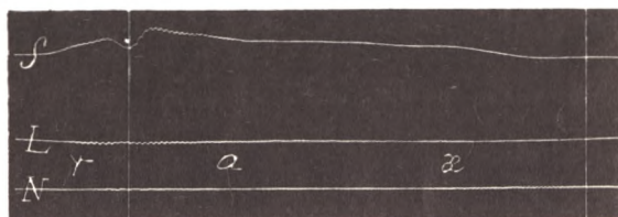
Фиг. 68. пая [gaæ].
