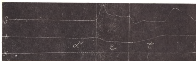
Фиг. 50. d'td\sigma [d'et].
