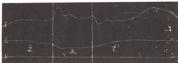
Фиг. 53. жатъ [zat'].
