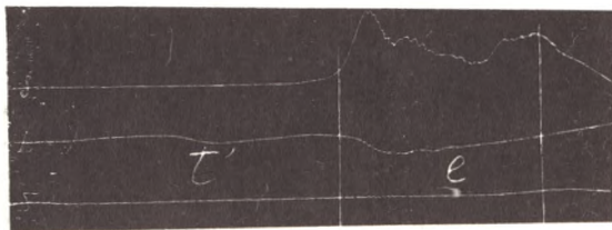
Фиг. 51. mъ [t'e].
