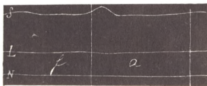
Фиг. 58. фа [fa], см. таблицу IV.
