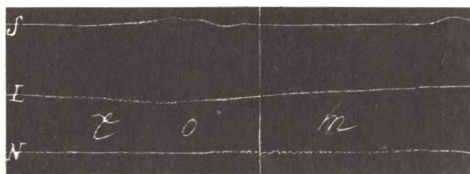
Фиг. 57. ломъ [lom].
