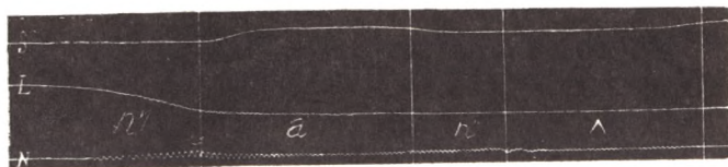
Фиг. 35. Няня [n'an'ɐ].
