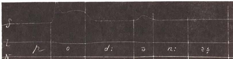
Фиг. 70. подданный [pod: ɐn : ɐ̃].
