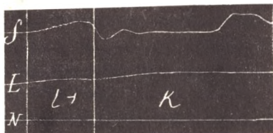
Фиг. 48. икѣ [l—k]
