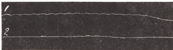
Фиг. 30. 1 — конецъ [u] въ утро ; 2 — конецъ [u] въ путь (тамбуринъ со слудой). Скорость 712 мп. въ 1". Увелич. почти въ 1.5.
