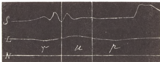
Фиг. 61. рубѣ [rup].
