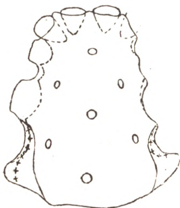
Фиг. 38. Сплошная линія — [ы]; крестиками — [ə].
